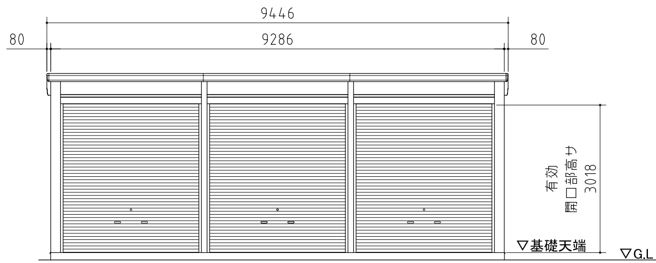
正面図
